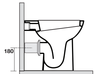
raccordo di scarico a parete art. 7539 connector for wall outlet art. 7539
