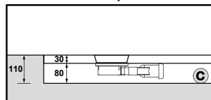
installazione filo pavimento floor level shower tray
