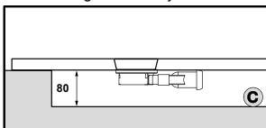
installazione in appoggio free standing shower tray
