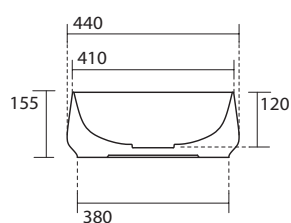
vista laterale
